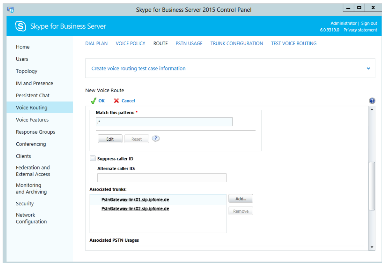
Abbildung 35: Alternative Rufnummer abgehend eingeben
