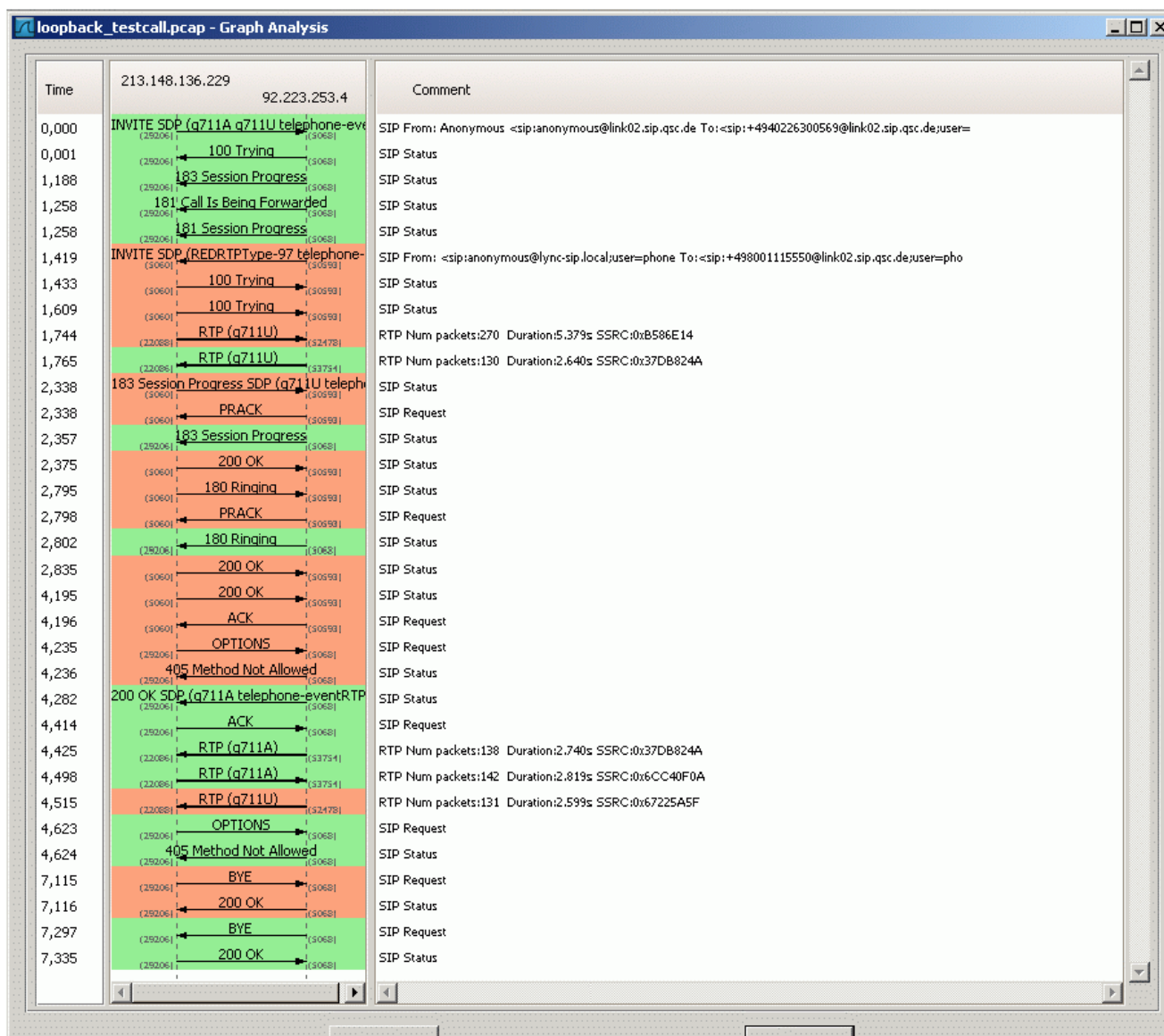
Abbildung 45: Grafische Wireshark-Analyse eines erfolgreichen Calls
