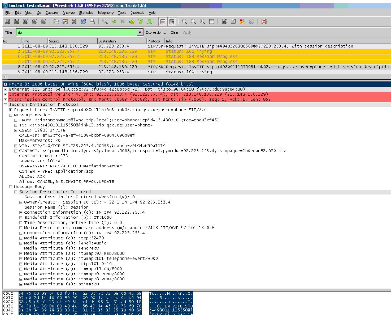
Abbildung 46: Grafische Wireshark-Analyse eines erfolgreichen Loopback-Tests
